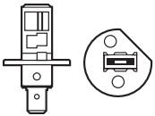
P14,5s IEC 7004-46
